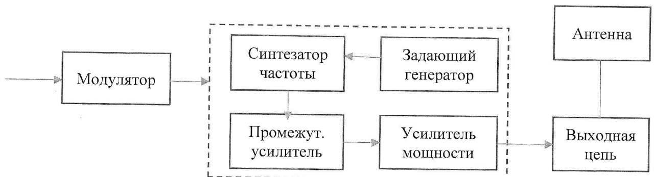
Рисунок 1 – Функциональная схема радиопередатчика
